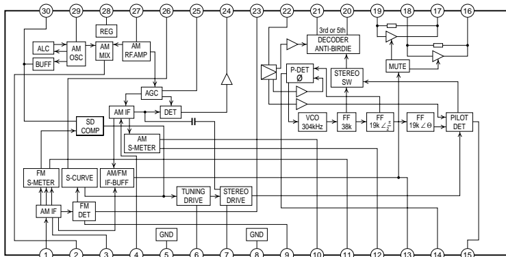
IC01 (LA1837)
