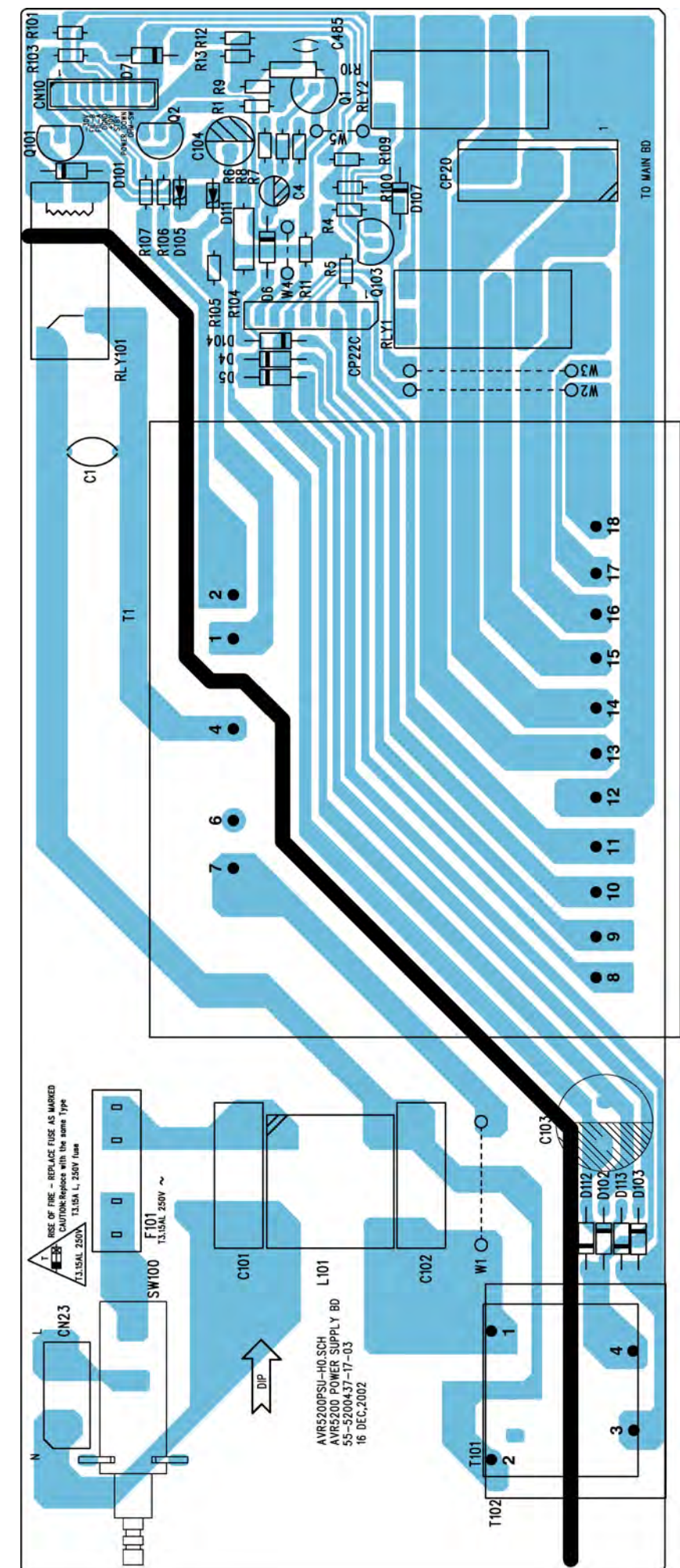
Sicht auf Bestückungsseite / View on Component Side
