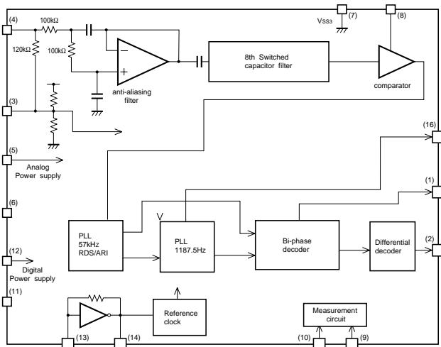
IC03 (BU1924F)
